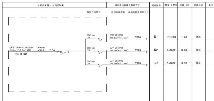
XXXXX 摊位配电系统图
